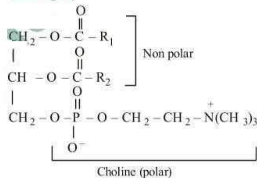
Fig. : Lecithin.
